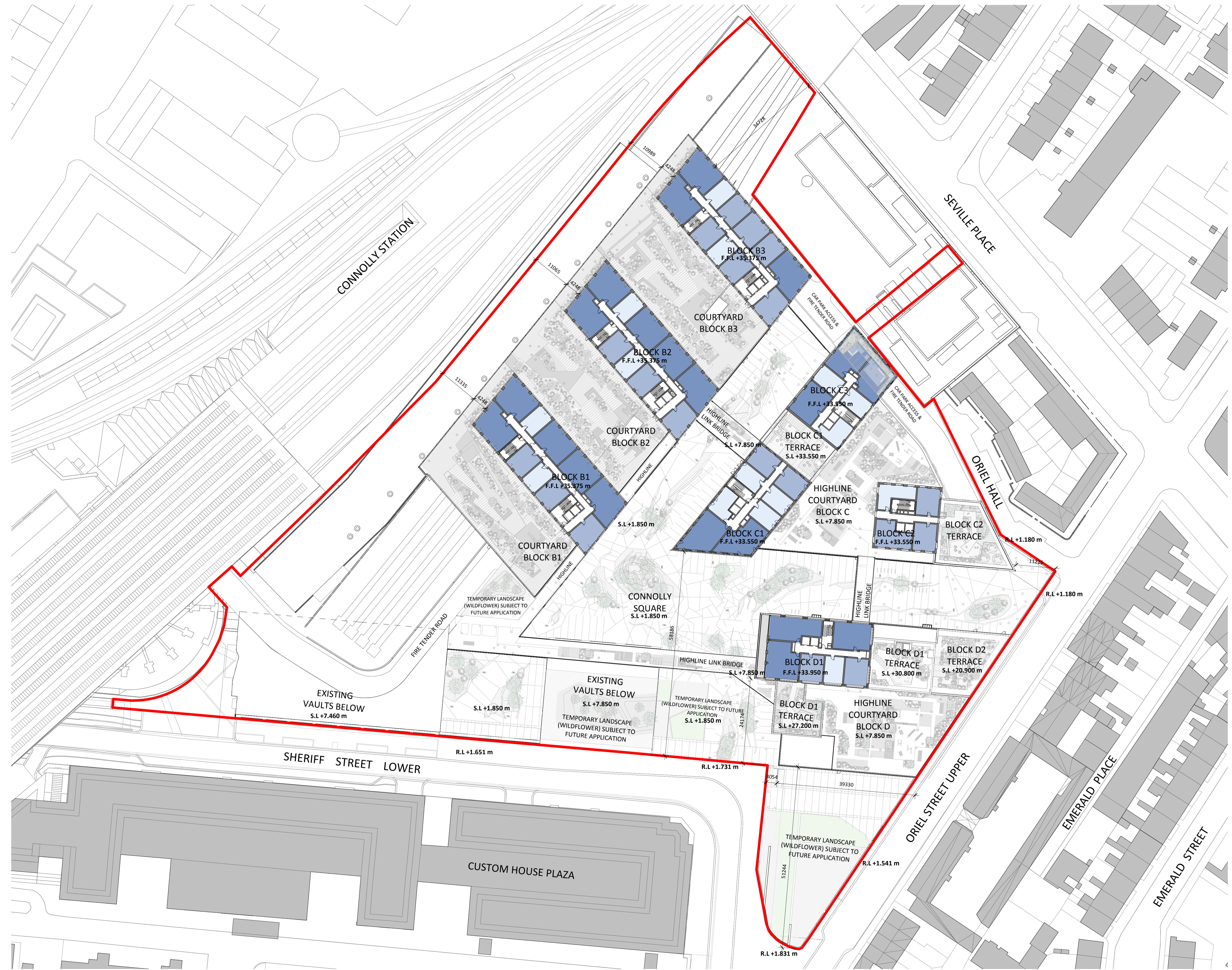
1 SITE LAYOUT PLAN - LEVEL 09 1 : 500
